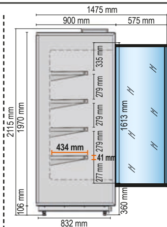
STROMBOLI 90 - C Spalle cieche / Blind side walls C Carne preconfezionata Pre-packed meat
