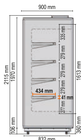
STROMBOLI 90 - C Spalle cieche / Blind side walls C Carne preconfezionata Pre-packed meat
